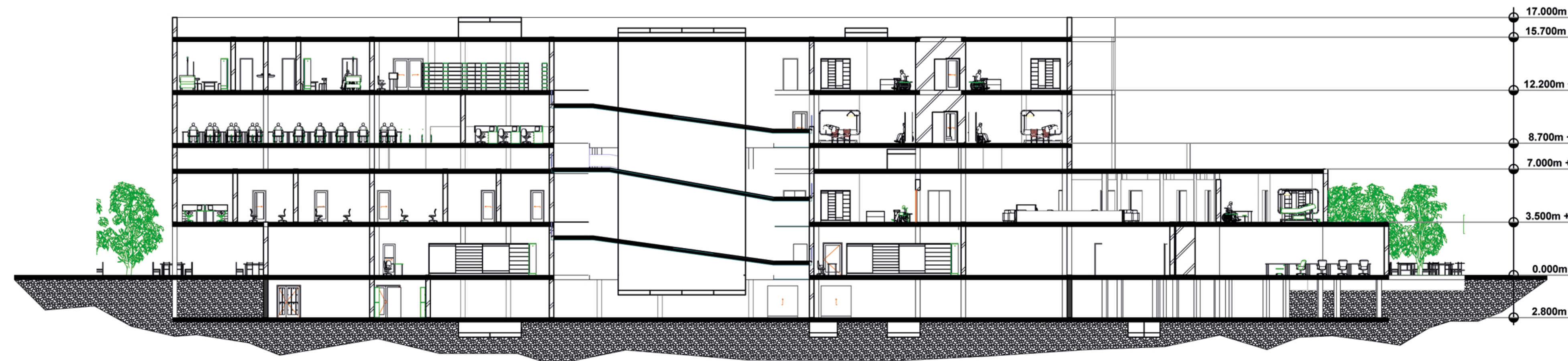
Section A-A
