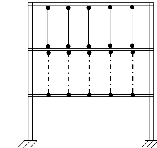
(d) Step 8 : Installation of Reshores Under Level 2
