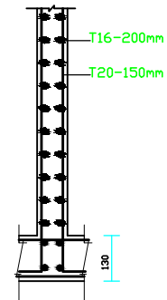
SECTION A-A
