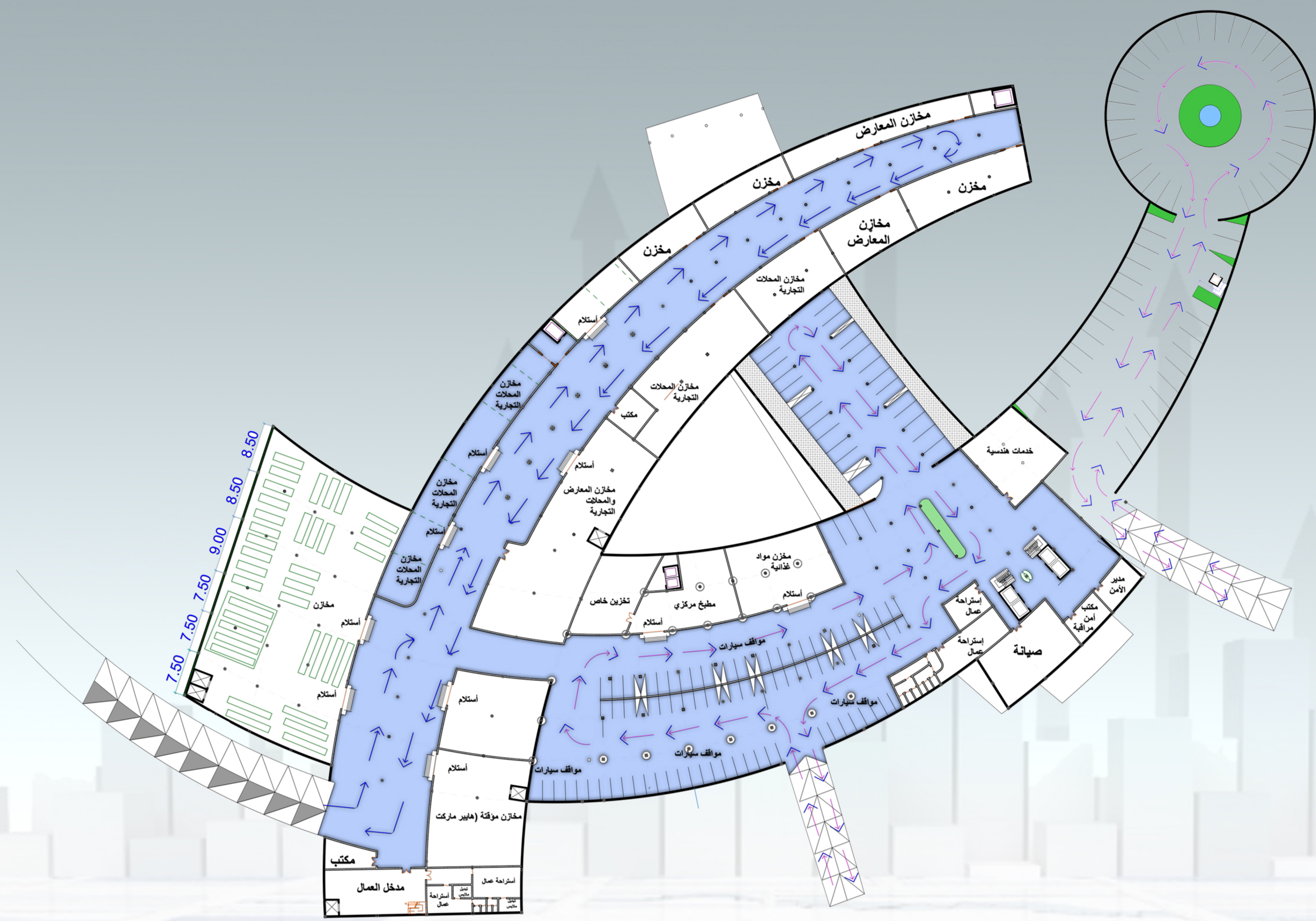
المسقط الأفقي للطابق تحت الأرضي مقياس الرسم 1:300
