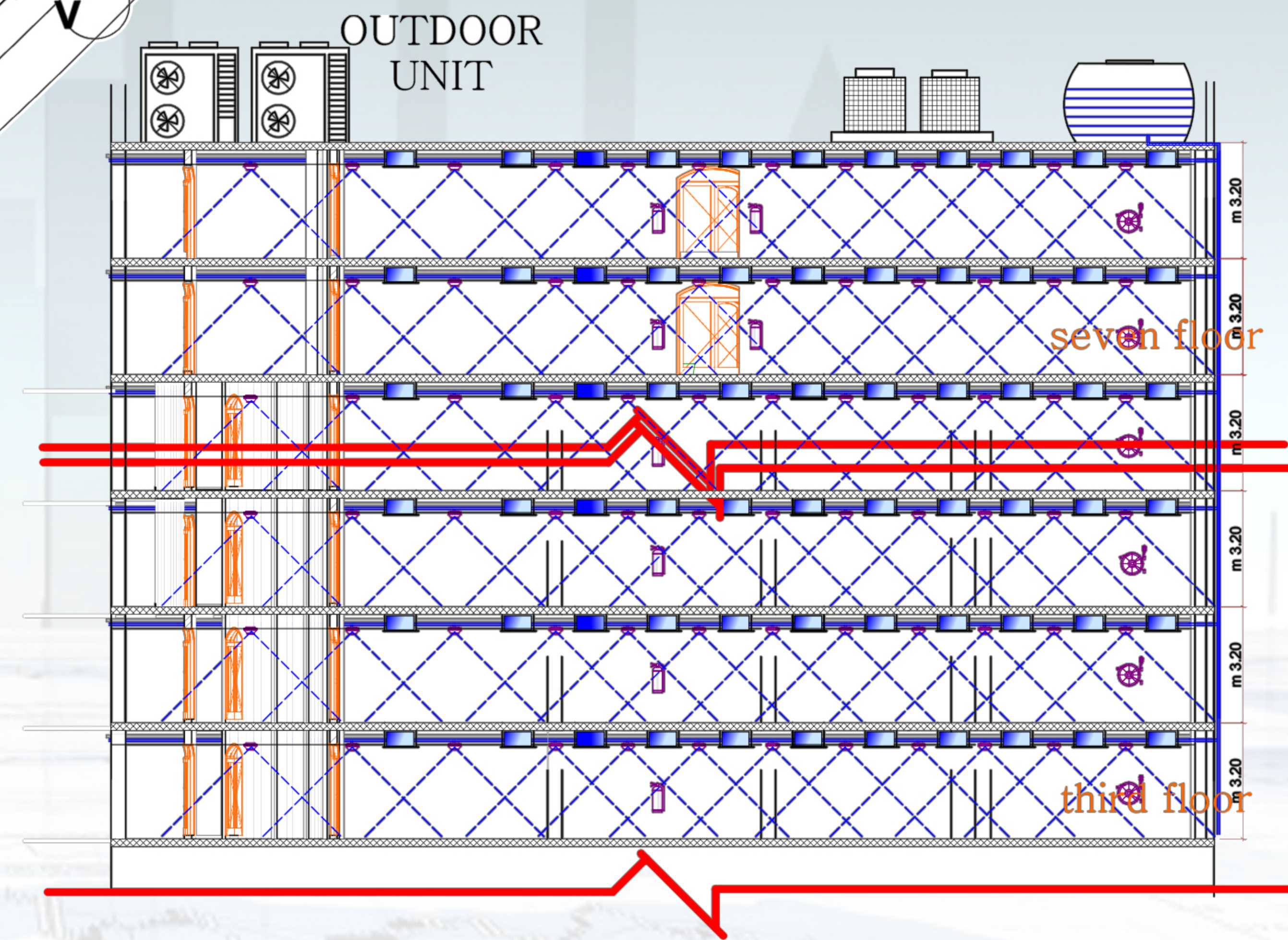
مساقط تفصيلية - أنظمة التكييف والحريق مقياس الرسم 1:100
