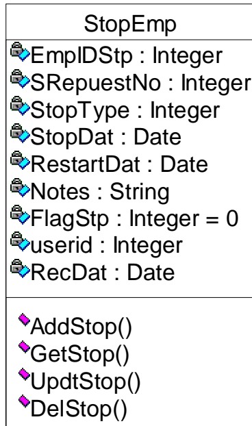
شکل ب.22: Stop Class
