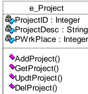
شکل ب.10: Project Class
