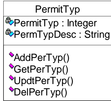
شکل ب.19: Permit Type Class
