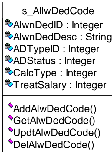
شکل ب.33: Allowances Class
