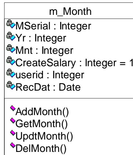
شکل ب.37: Month Class
