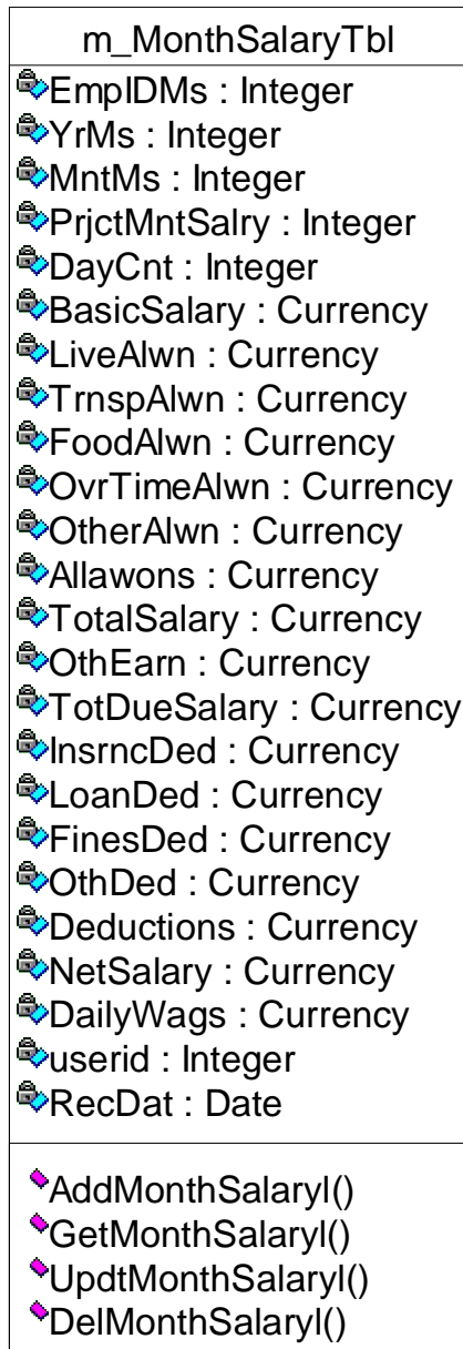
شکل ب.38: Month Salary Class
