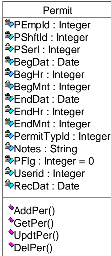
شکل ب.20: Permit Class
