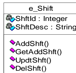
شکل ب.13: Shift Class
