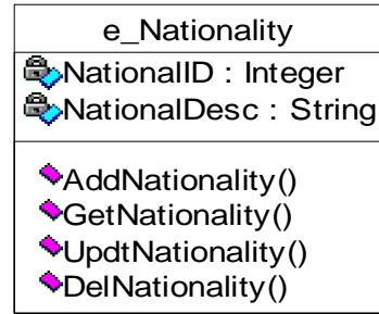
شکل ب.7: Nationality Class
