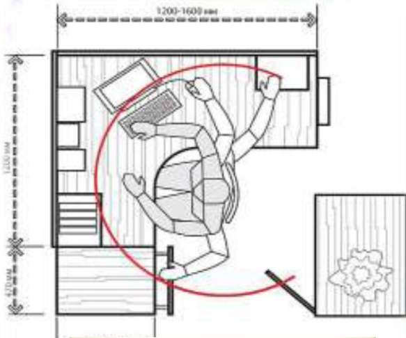
الرسمه 45 توضح مكاتب الموظفين
