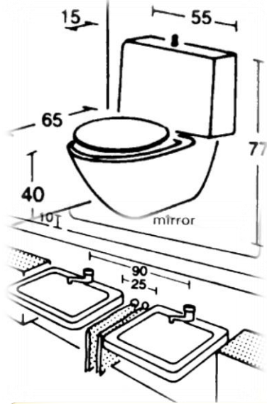
الرسم 40 توضح ابعاد المراض والمغاسل
