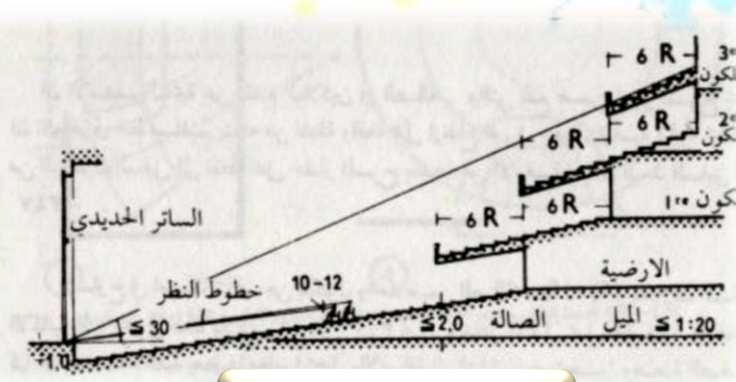
الرسم 22 توضح خط النظر
