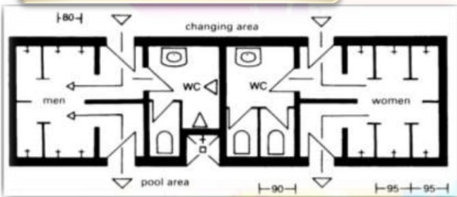
الرسمه 33 توضح غرف تخديم المسبح
