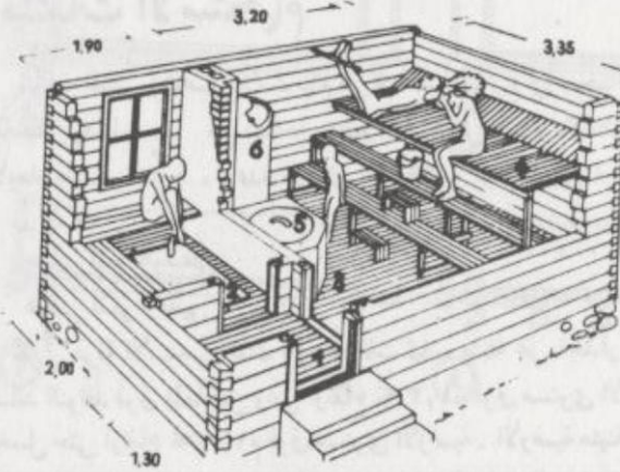
الرسمه 34 توضح ابعاد غرفة الساونا
