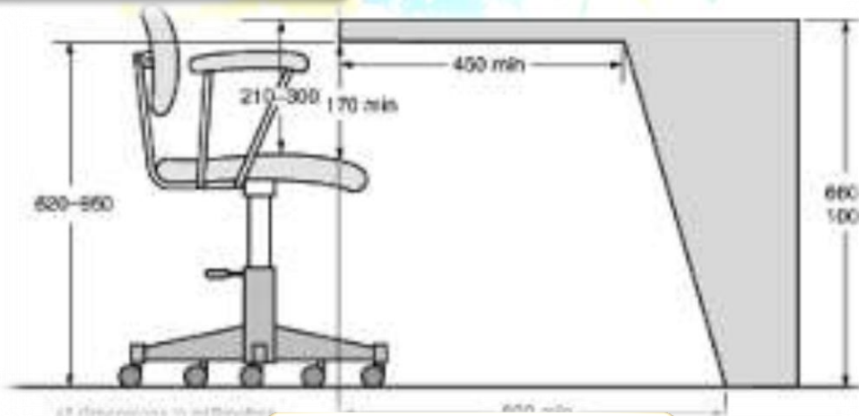
الرسمه 46 توضح ابعاد المكتب
