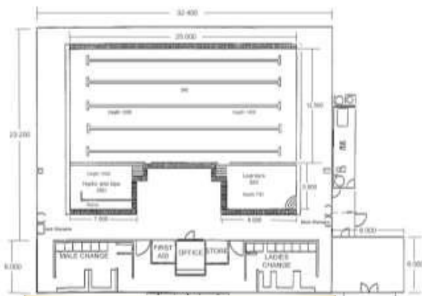
الرسمه 32 توضح ابعاد المسبح
