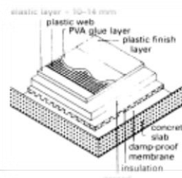
الرسم 30 توضح تفاصيل أرضية ألعاب القوى
