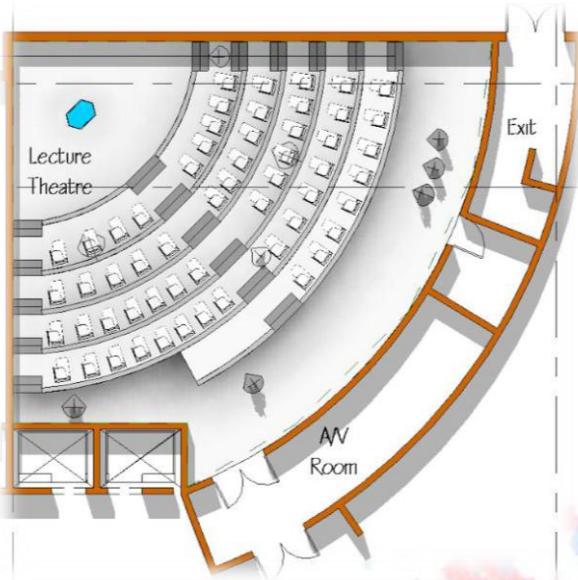
الرسم 15 توضح مسقط افقي بقاعة تدريبية
