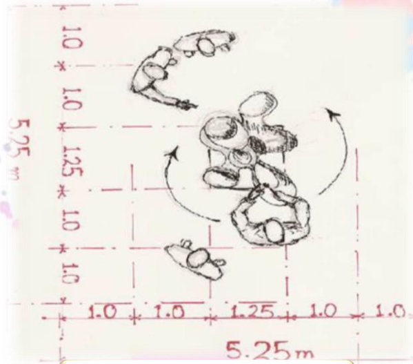
الرسمه 14 توضح ابعاد طاولة النحت
