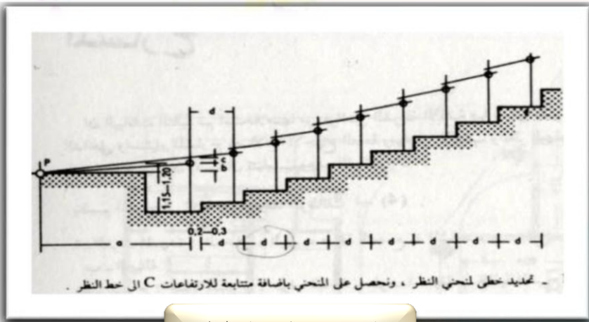
الرسم 21 توضح خط النظر
