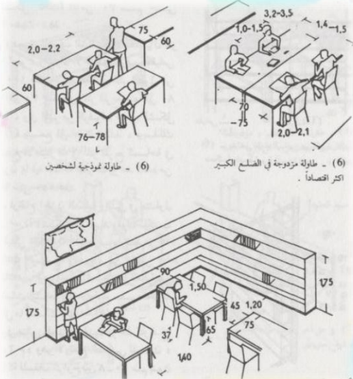
الرسم 16 توضح ابعاد الجلسات المكتبية
