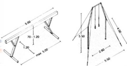
الرسم 29 توضح ابعاد لجة الجينازيوم
