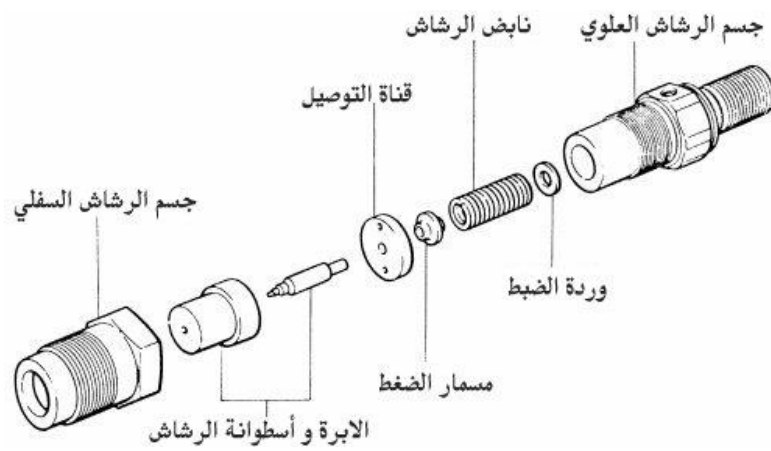
الشكلين (5-27) ترتيب أجزاء الرشاش
