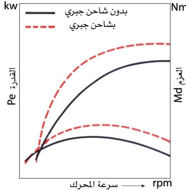
شكل (5-4) يوضح العزم والقدرة في حالة استخدام شاحن جبري او بدونه
