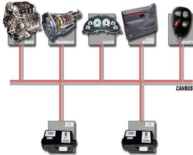
شكل (4-23) يوضح أنظمة الربط
