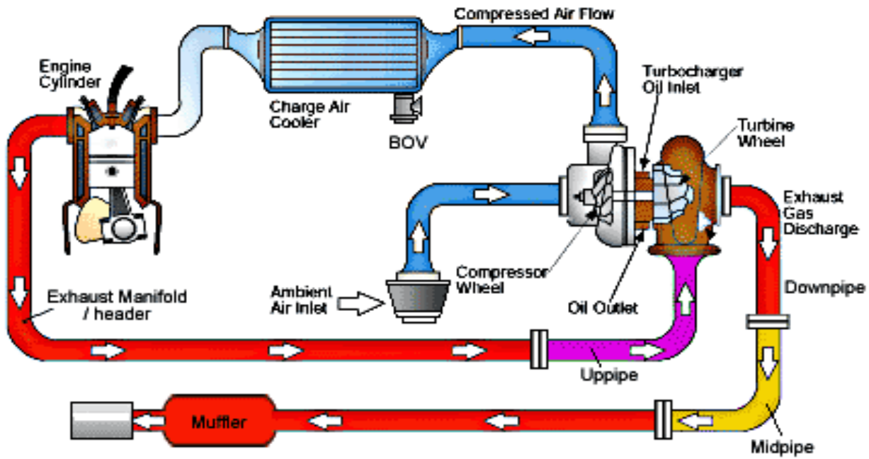
شكل (8-4) يوضح طريقة عمل التيربو تشارجر
