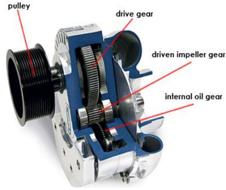
الشكلين (11-4) نوعين من الشاحن الميكانيكي Super charger
