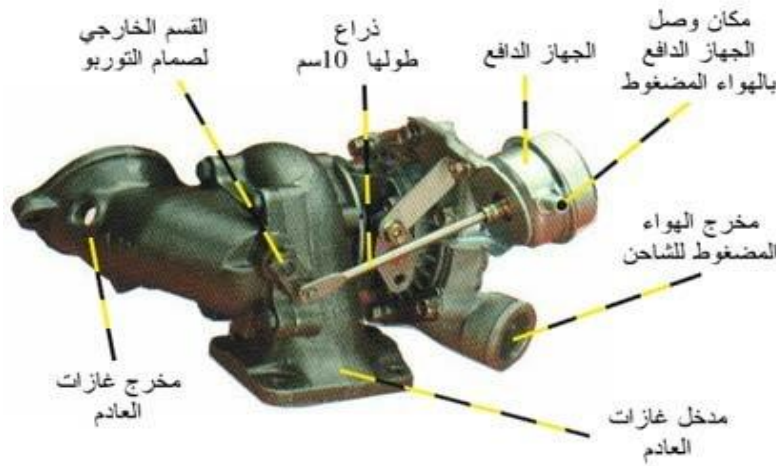
شكل (1-4) الأجزاء الخارجية لشاحن الهواء التوربين
