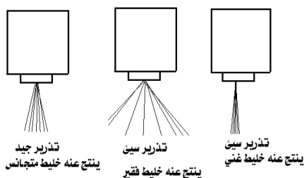
الأشكال (32-5) أشكال التذرية عند عمل رشاش الديزل
