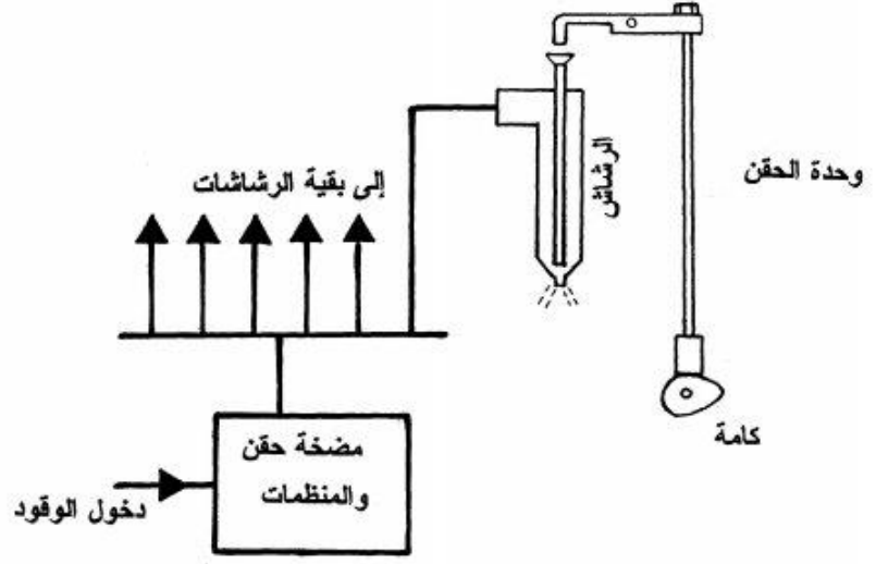
شكل (2-6) مخطط لنظام حقن ديزل بوحدة حقن مفصلة
