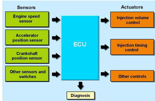
الشكل (4-25) يوضح المدخلات والمخرجات في وحدة ECU
