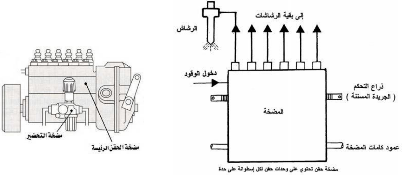
شكل (4-2) مخطط لنظام حقن ديزل بمضخة مستقيمة
