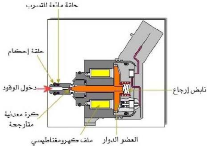
الشكلين (3-8) يبين شكل وأجزاء صمام التحكم بضغط الوقود
