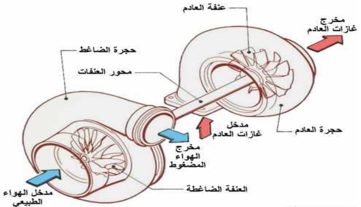
شكل (4-13) يوضح تصميم التيربو
