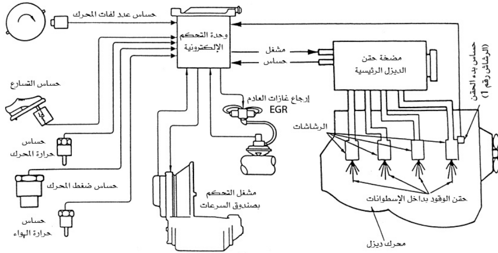
شكل (2-7) مخطط لنظام حقن ديزل بتحكم كهربائي
