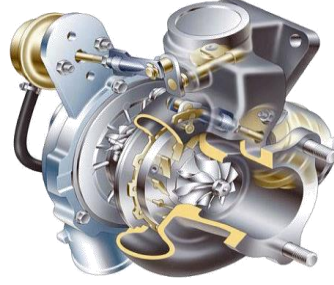
شكل (4-4) يوضح التيربو من الداخل
