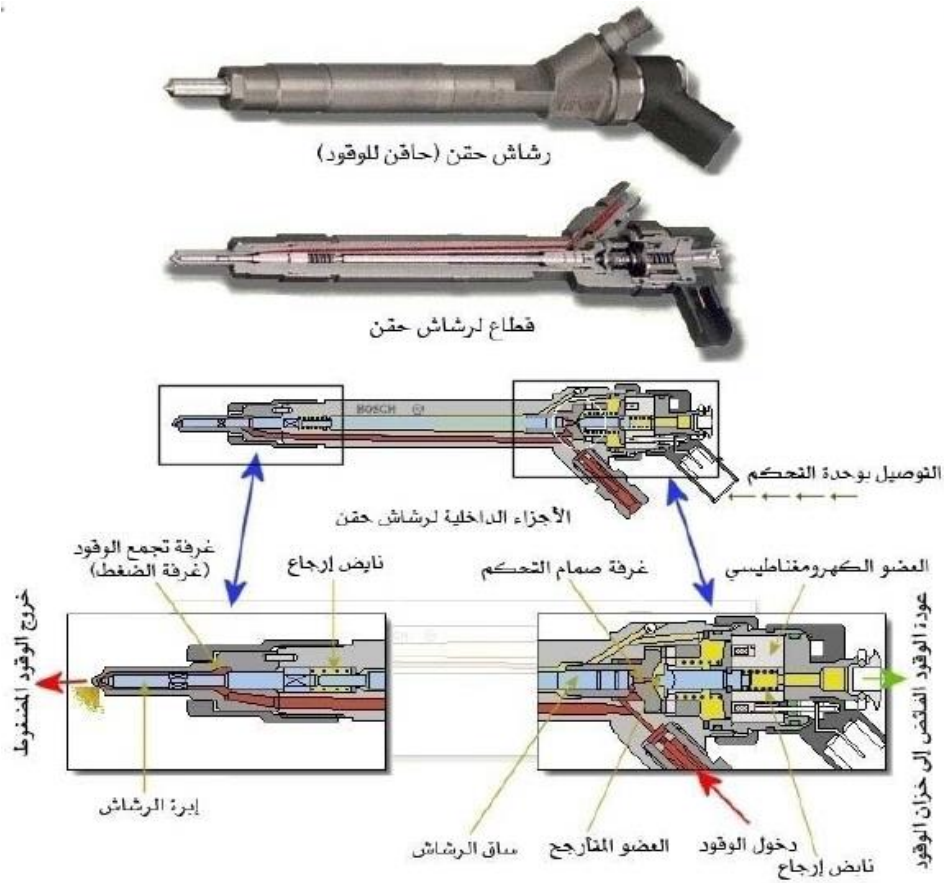
الأشكال (3-11) يبين الشكل الخارجي والأجزاء الداخلية للرشاش
