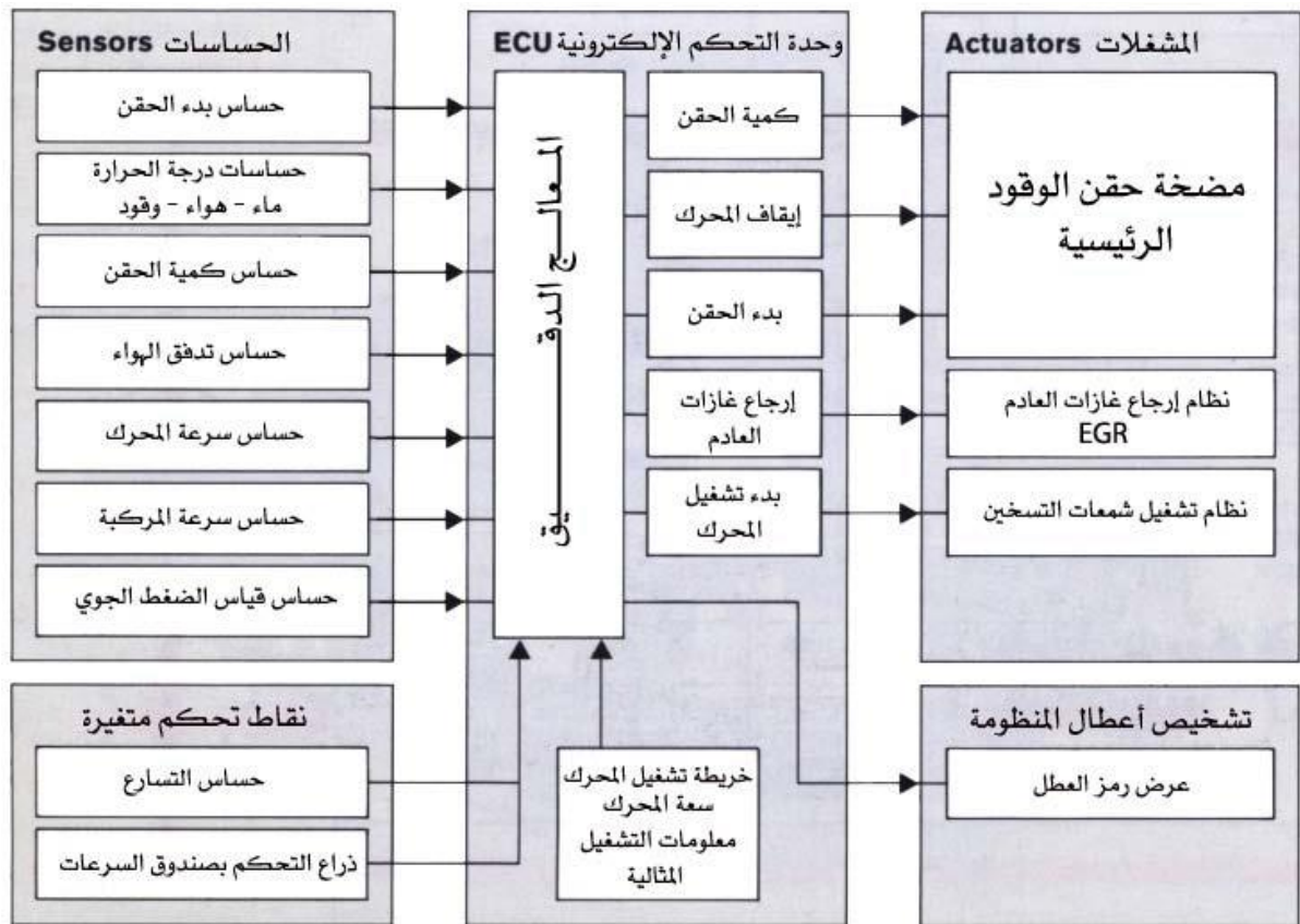
شكل (4-29) يبين مخطط منظومة حقن الديزل بتحكم إلكتروني وأجزائه الأساسية
