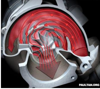
شكل (4-4) يوضح التيربو من الداخل
