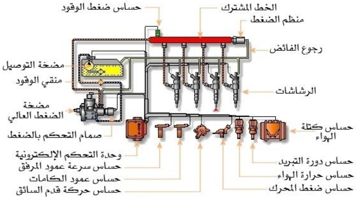
الشكل (3-14) يبين أجزاء النظام بالتفصيل
