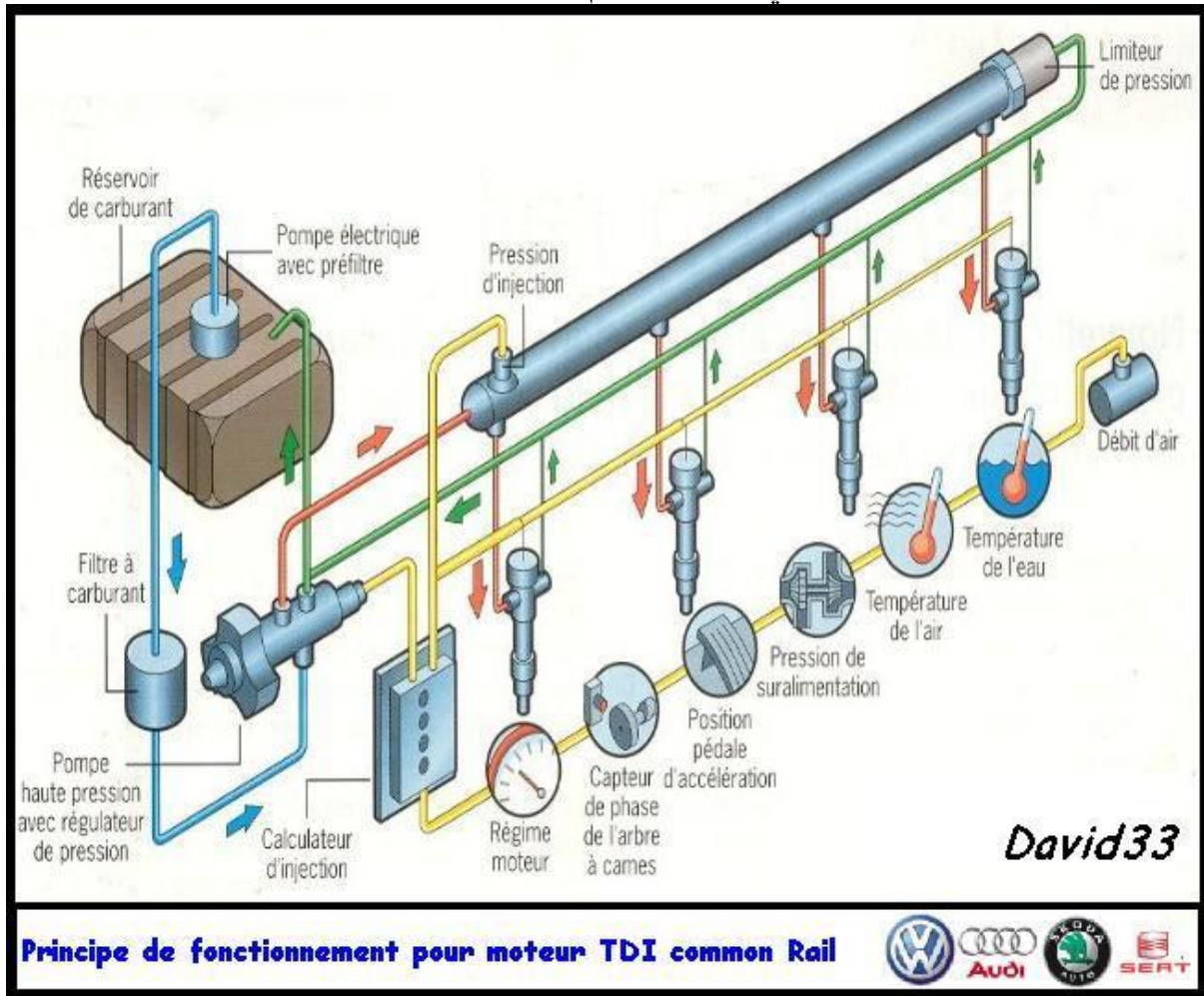
الشكل (2-15) أجزاء TDI Common Rail
