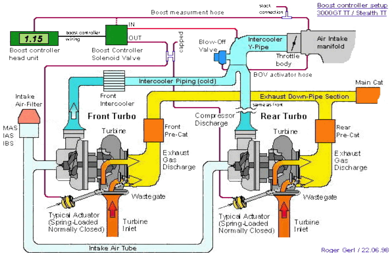
شكل (12-4) Twin turbo
