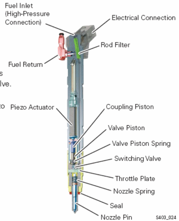
الشكل (3-12) مخطط رشاش TDi
