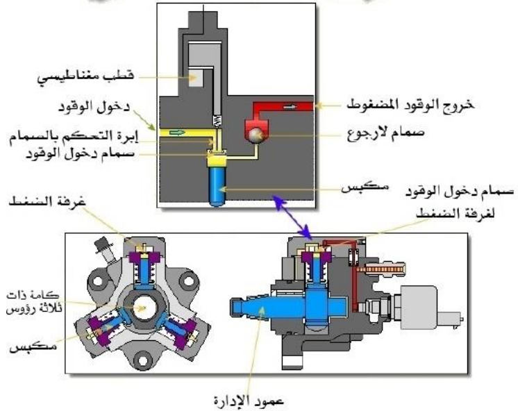
الأشكال (3-7) يبين أجزاء مضخة الضغط العالي
