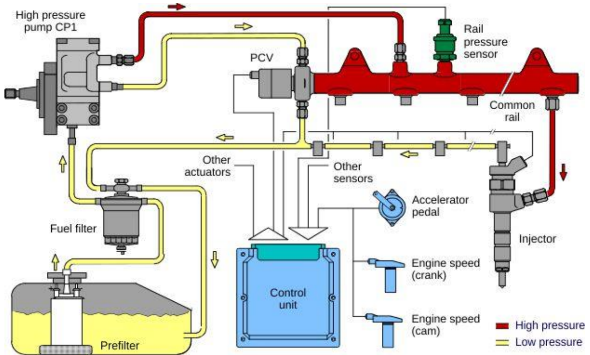
الشكل (3-4) مسميات أجزاء نظام الأنبوب المشترك
