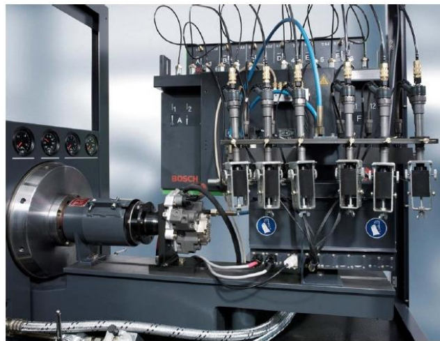
شكل (5-19) جهاز فحص الرشاشات
