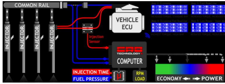
شكل (4-22) معالجة الإشارات وعمليات وحدة التحكم الإلكترونية
