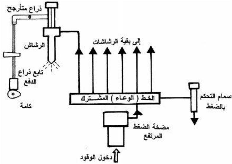
شكل (2-11) مخطط لنظام حقن ديزل بخط مشترك
