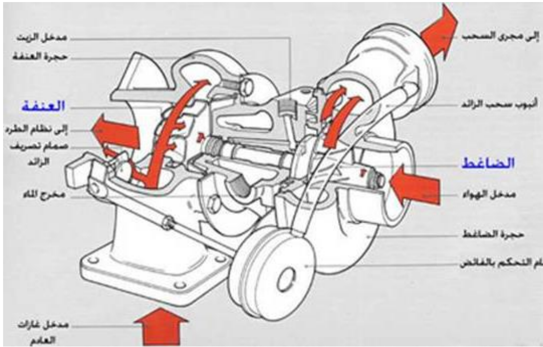
شكل (7-4) قطاع لأجزاء التيربو
