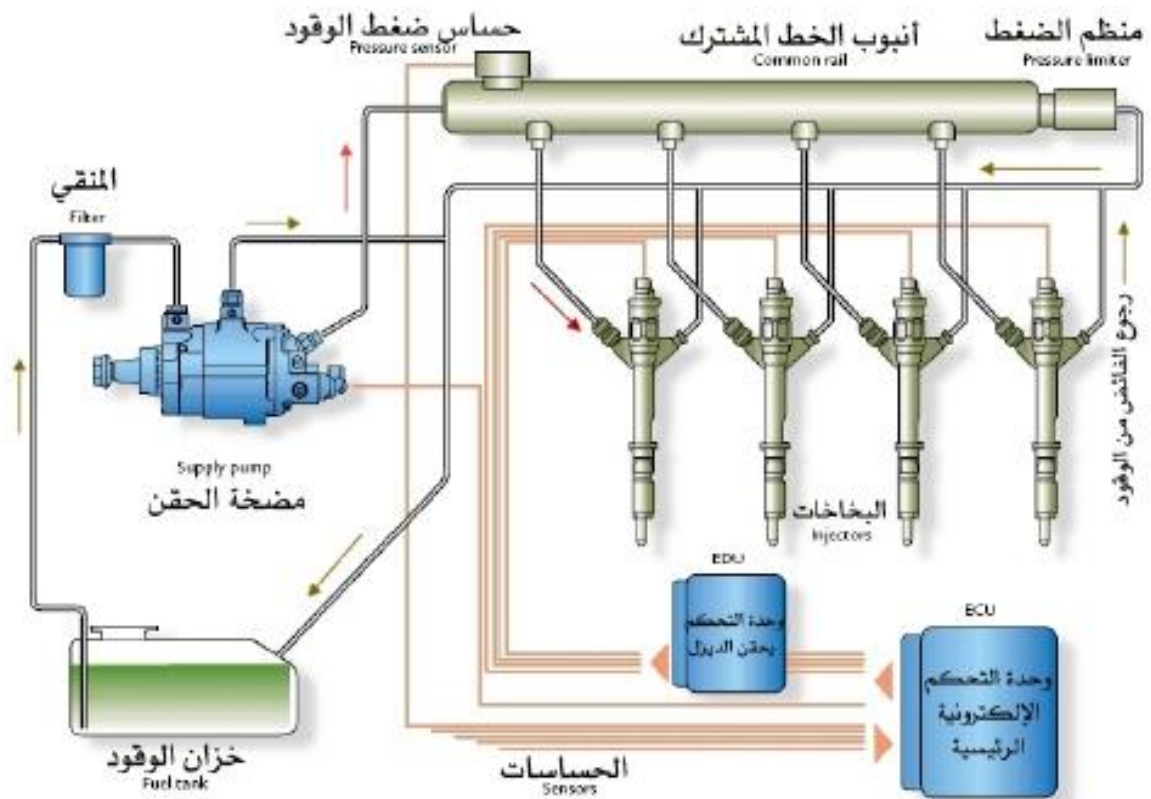
الشكل (3-4) مسميات أجزاء نظام الأنبوب المشترك
