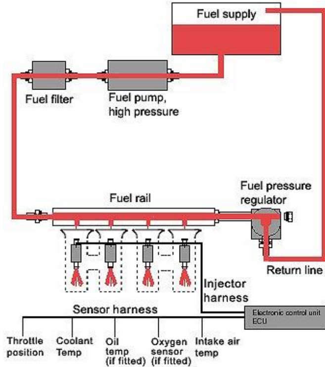
الشكلين (2-12) مخطط وأجزاء نظام حقن ديزل بخط مشترك تحكم إلكتروني
