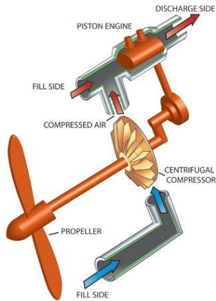
الشكلين (11-4) نوعين من الشاحن الميكانيكي Super charger
