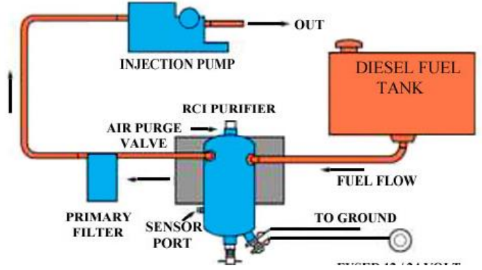
الشكل (3-13) الأجزاء الأساسية لأنظمة حقن الديزل
