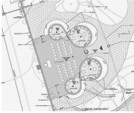
رسم هندسي رقم 2- 10 يوضح مسقط الصالة متعددة الاغراض
