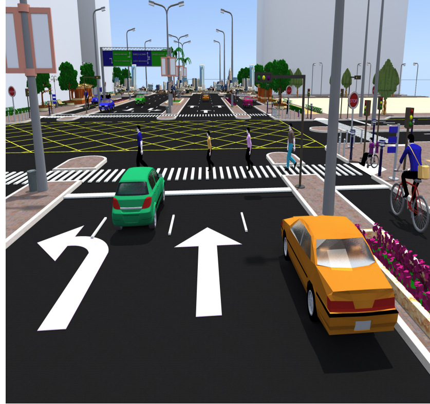
شكل (٥-١٣) منظور لمنطقة حارات السير عند التقاطع وعبور المشاة
