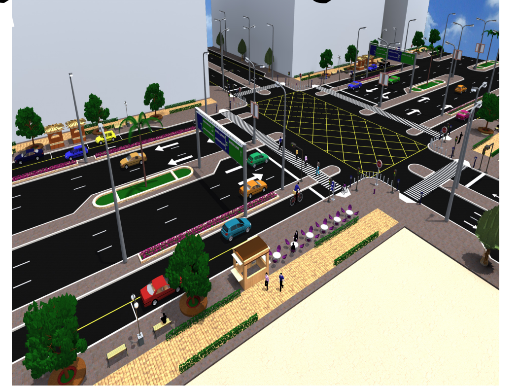
شكل (٥-١٢) منظور لمنطقة تقاطع شارع القصر مع شارع البلدية مع الرصيف الجانبي والجزر الوسطية
