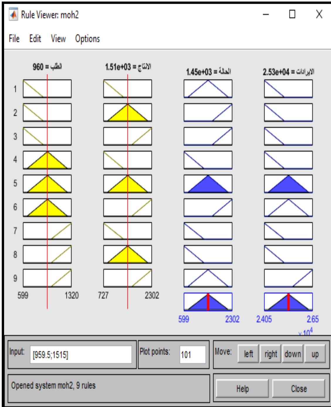
شكل (A3-4) عارض القاعدة (Rule Viewer) لمنتج النفط الابيض
