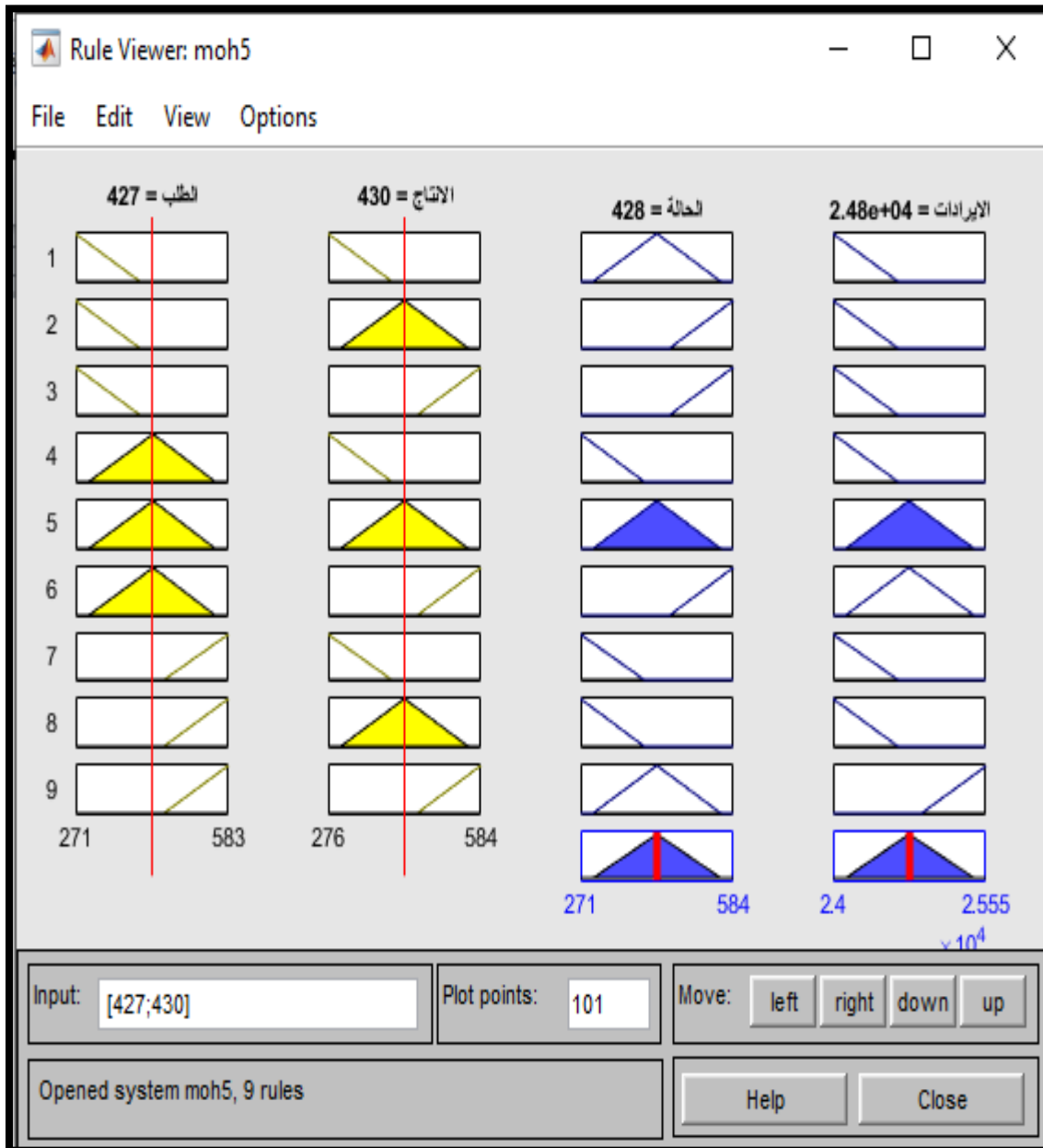
شكل (A18-4) عارض القاعدة (Rule Viewer) لمنتج زيت الديزل
