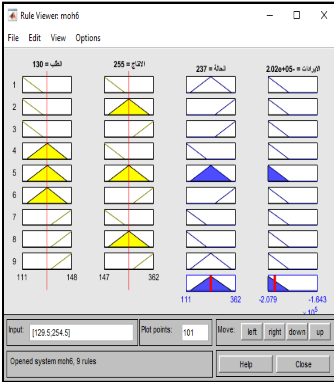
شكل (A28-4) عارض القاعدة (Rule Viewer) لمنتج الغاز السائل
