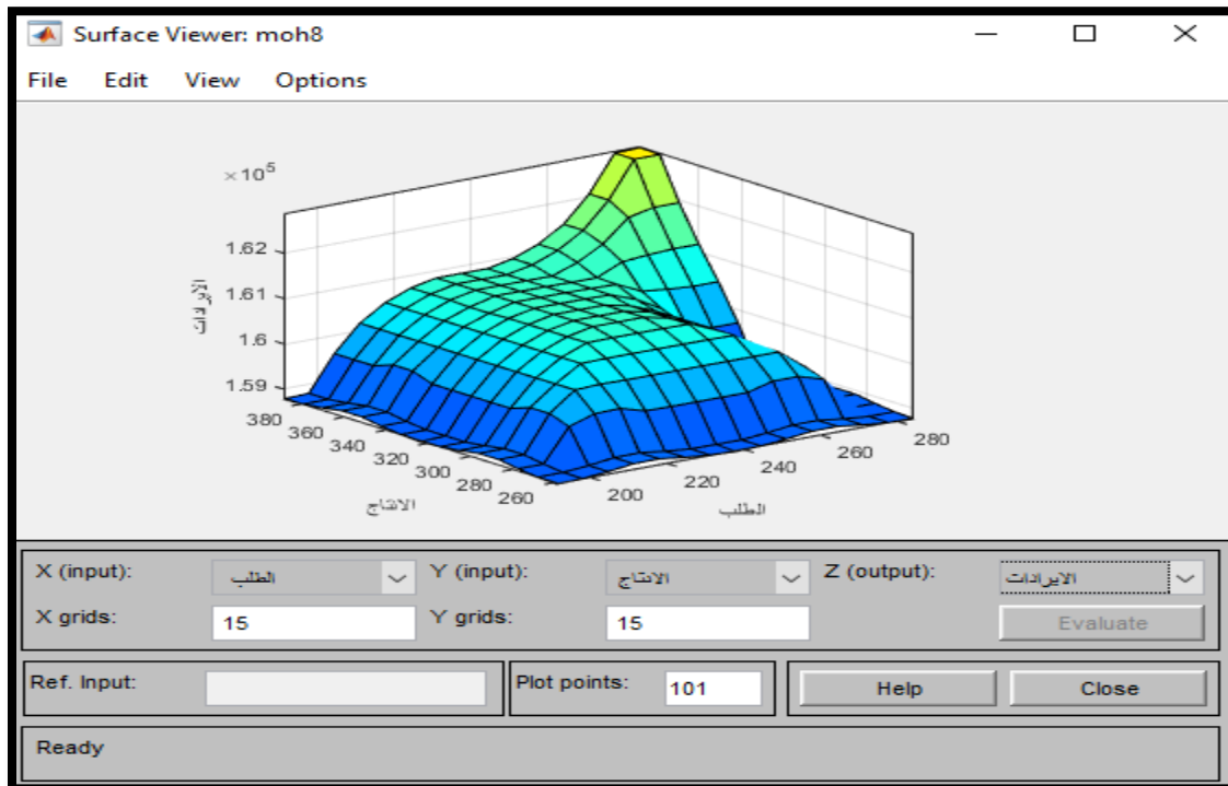
شكل (A10-4) يمثل عارض السطح (Surface Viewer) حسب الايرادات لمنتج وقود طائرات
