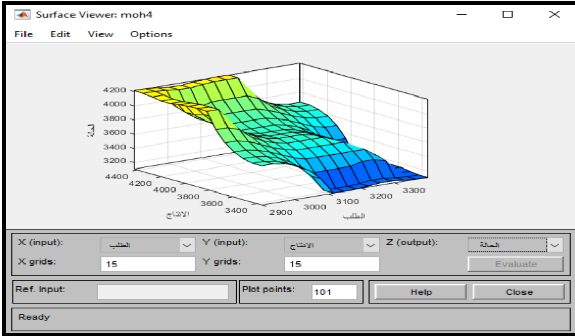
شكل (A15-4) يمثل عارض السطح (Surface Viewer) حسب الايرادات لمنتج زيت الغاز
