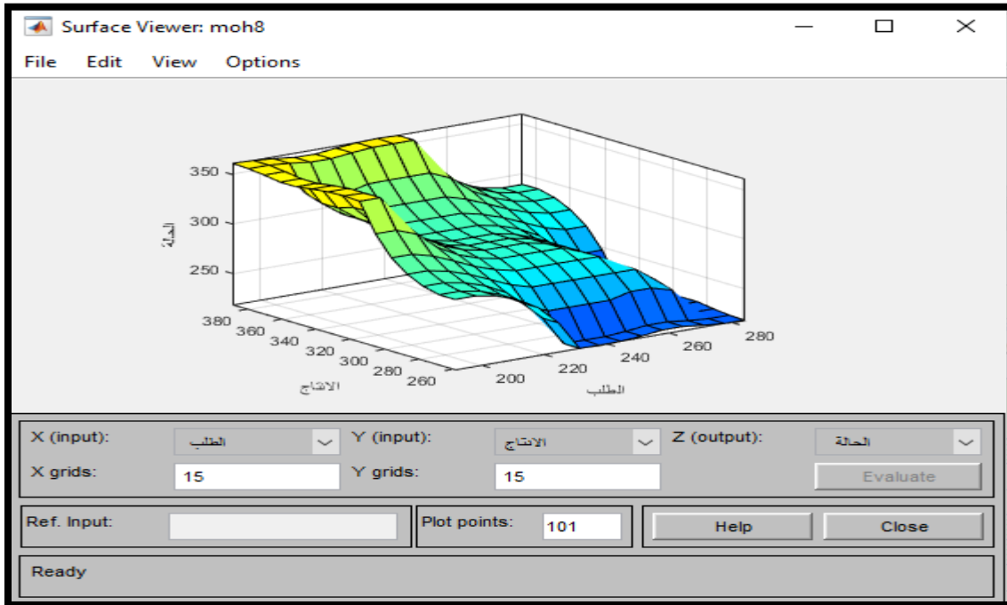
شكل (A9-4) يمثل عارض السطح (Surface Viewer) حسب الحالة (كمية الخزين) لمنتج وقود طائرات
