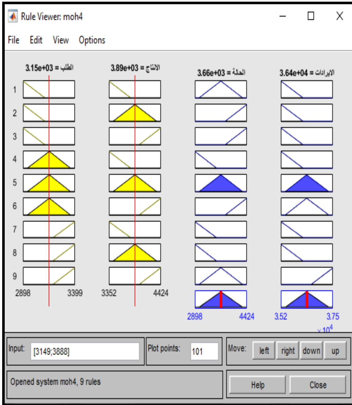
شكل (A13-4) عارض القاعدة (Rule Viewer) لمنتج زيت الغاز
