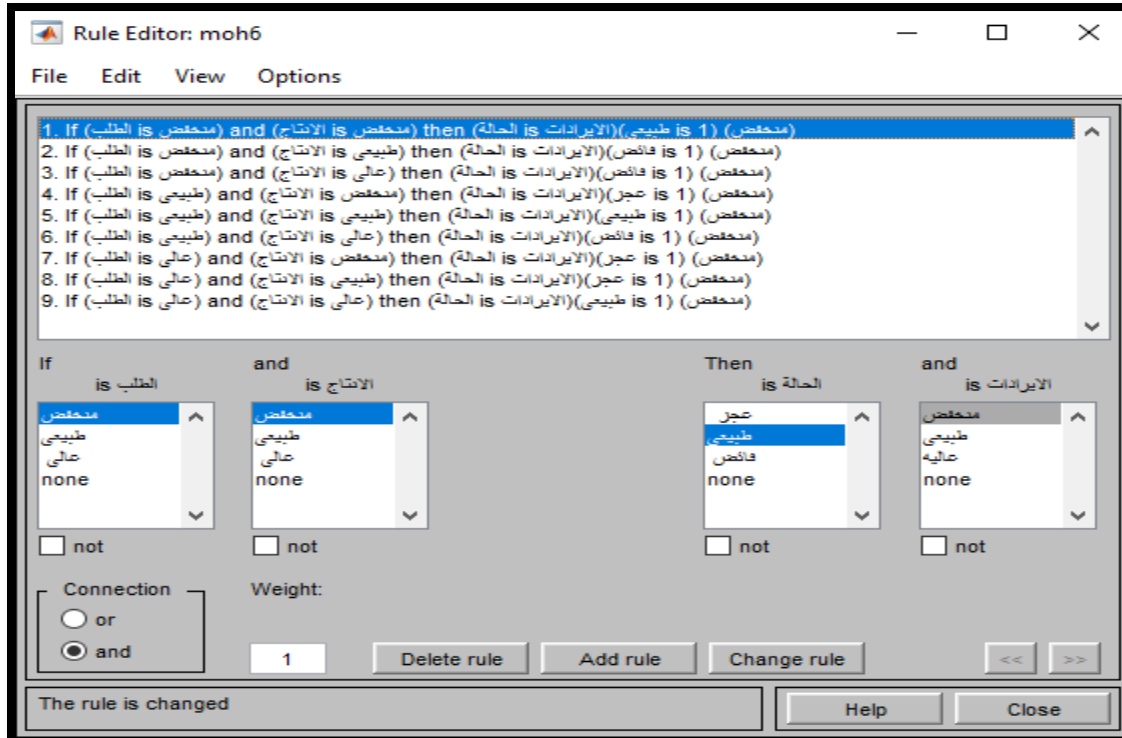
شكل ( A27-4 ) محرر القواعد (Rule Editor) لنظام الاستدلال الضبابي (FIS) لمنتج الغاز السائل
