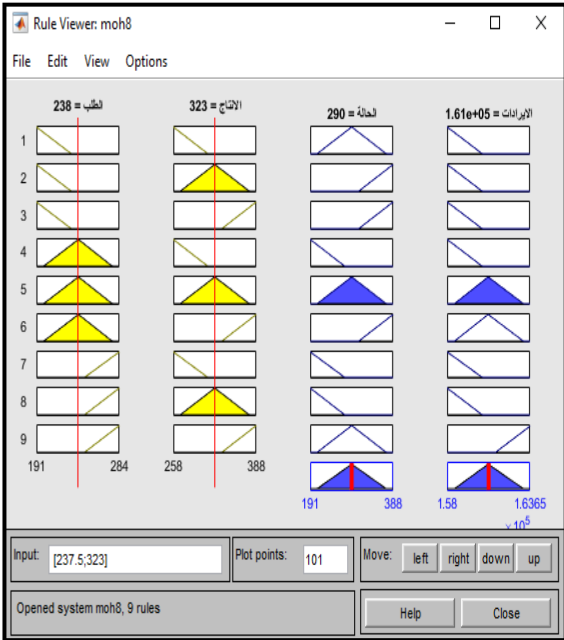
شكل (A8-4) عارض القاعدة (Rule Viewer) لمنتج وقود طائرات
